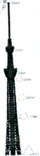
東京スカイツリーの作図されたシルエット(影)と地上が正三角形(1辺68m)で次第に丸くなり、地上約320mでほぼ真円となる断面[20]
